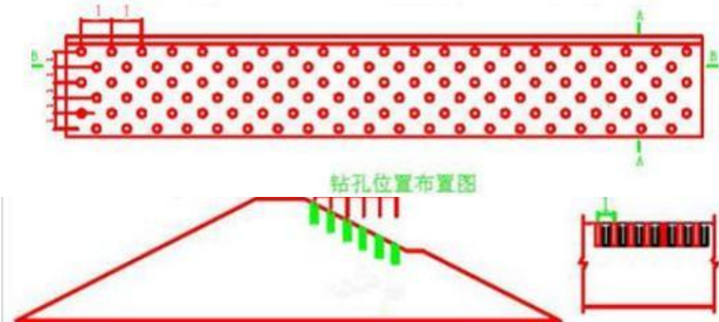
A-A(孔深 2 米)B-B(孔距 1 米)
